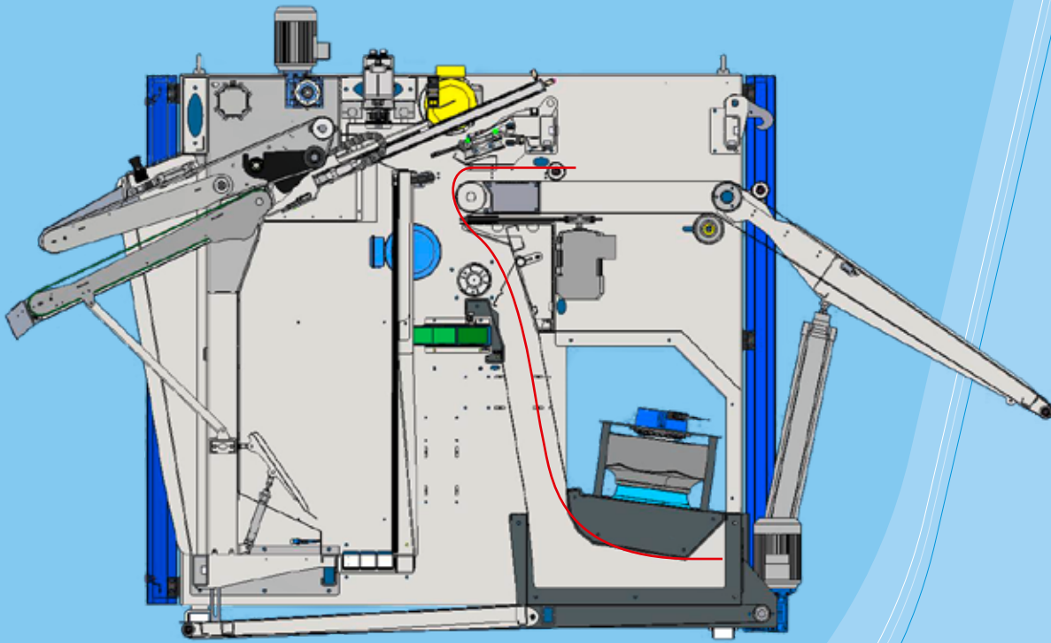
Schéma de principe montrant la nouvelle Jenfeed Express Plus incorporant la nouvelle trappe d'aspiration permettant de traiter les draps grande taille.
